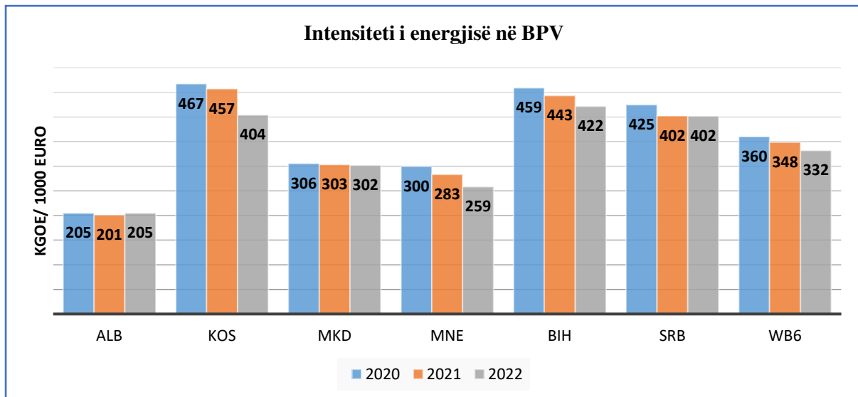
Figura 11: Intensiteti i energjisë
